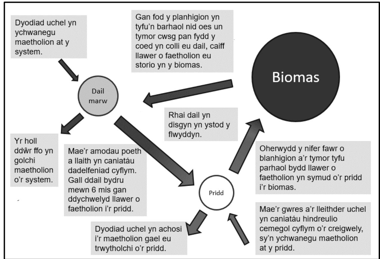
Ffigur 1. Y gylchred faetholion mewn coedwig law drofannol
